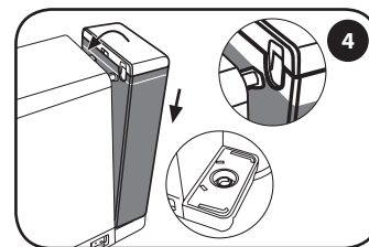
4 Reinscrivere il serbatoio in corrispondenza delle due fessure e accompagnarlo verso la macchina fino a completo aggancio. Controllare che il serbatoio sia completamente agganciato.
