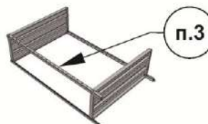
Рис.4 Наживить третью стойку п.3 винтами М5х16 п.4 к полкам п.2.
